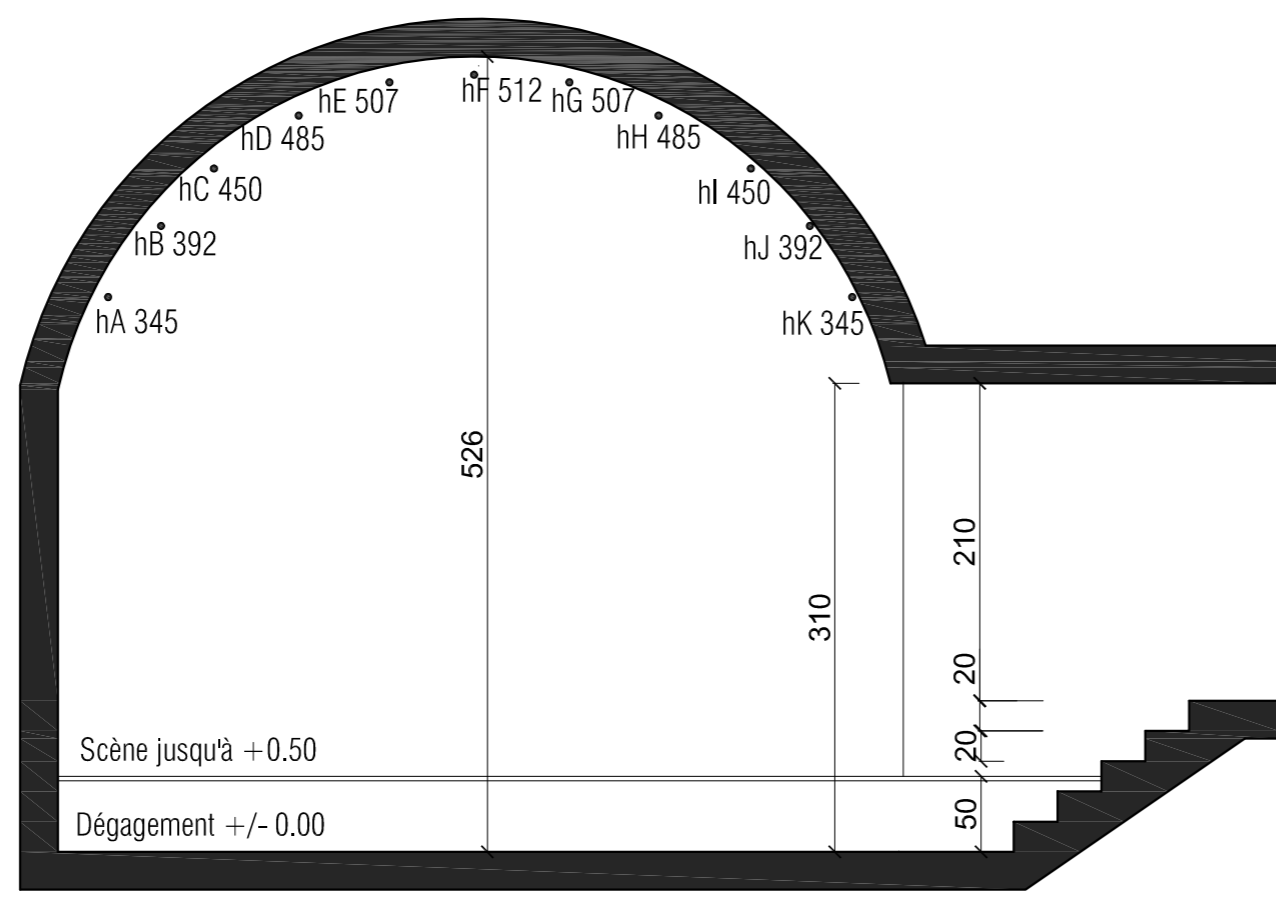
COUPE AA ( hauteurs données depuis le dégagement à ± 0.00 )
