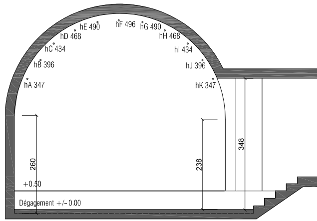
COUPE AA
